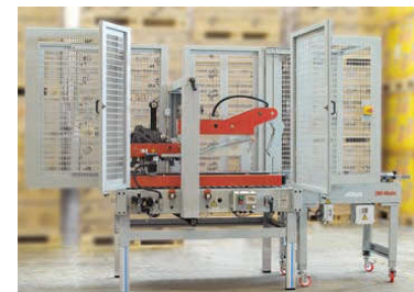
Vollautomatischer Kartonschleier
